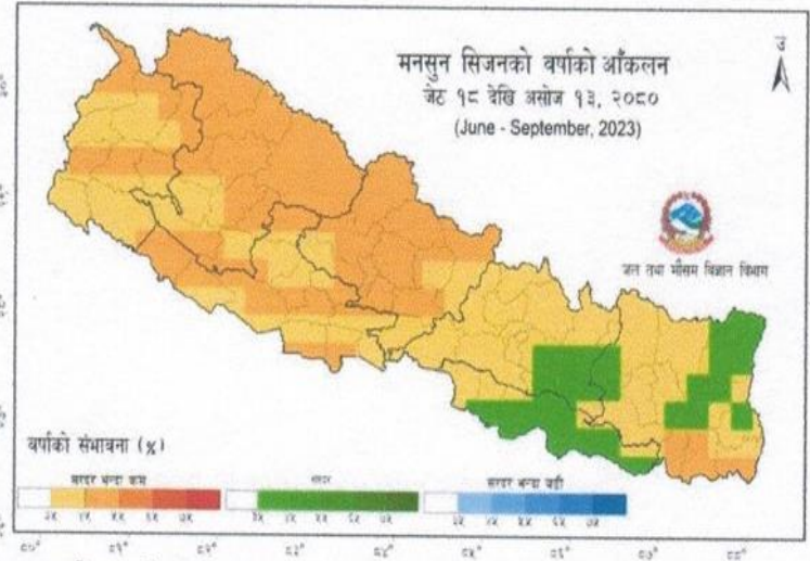
चित्र १: २०५० को मनसुन सिजनको वर्षा (सर्दर भन्दा कम वा सर्दर वा सर्दर भन्दा बढी) को सर्वाधिक सम्भावना (%)
