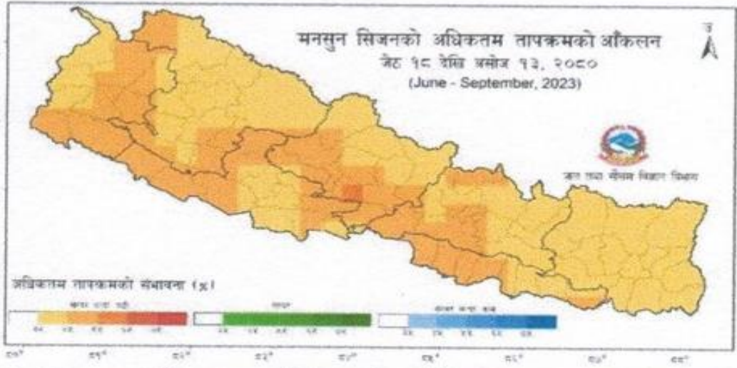
चित्र २: २०५० को मनसुन सिजनको अधिकतम तापक्रम (सर्दर भन्दा कम वा सर्दर वा सर्दर भन्दा बढी) को सर्वाधिक सम्भावना (%)
