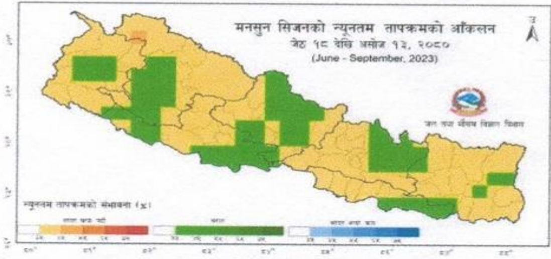
चित्र ३: २०५० को मनसुन सिजनको न्यूनतम तापक्रम (सर्दर भन्दा कम वा सर्दर वा सर्दर भन्दा बढी) को सर्वाधिक सम्भावना (%)
